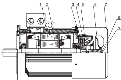
图1 电磁制动马达
